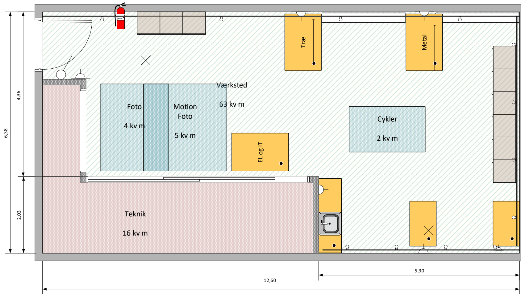
FORSLAG TIL INDRETNING AF KÆLDER Hjorteparken- Kælderplan 1:50
